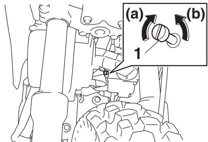
1. Leerlaufeinstellschraube
